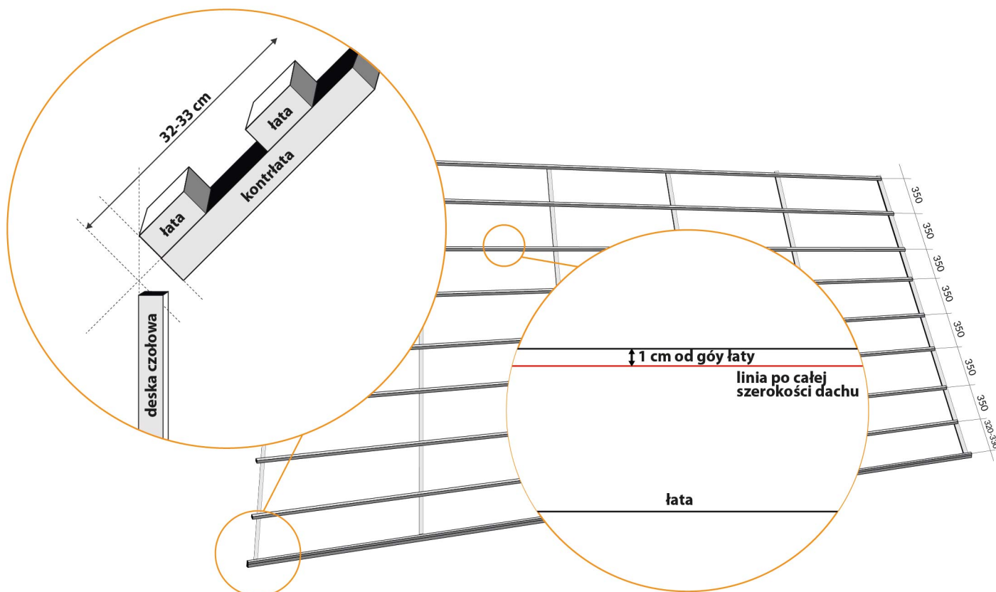
Montaż do łąt i kontrłąt
